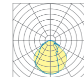
Asymmetrische Abstrahlung
